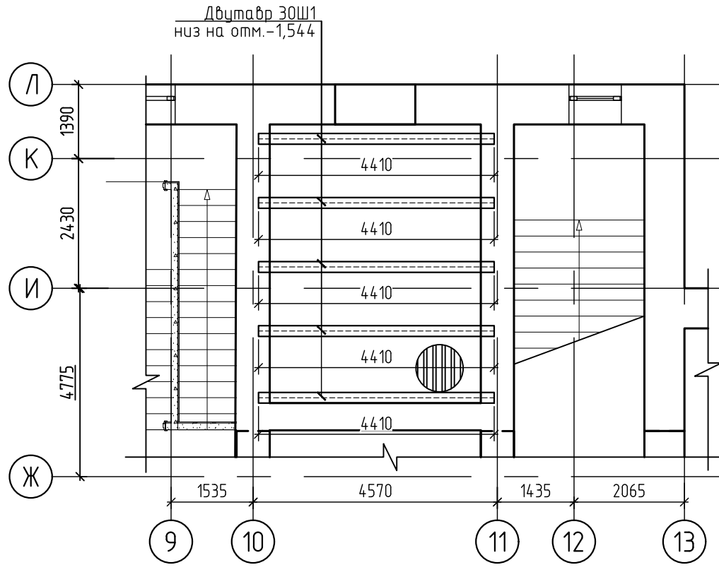
Схема расположения металлических балок перекрытия в осях 9-11 / Ж-Л на отм. -1,050
