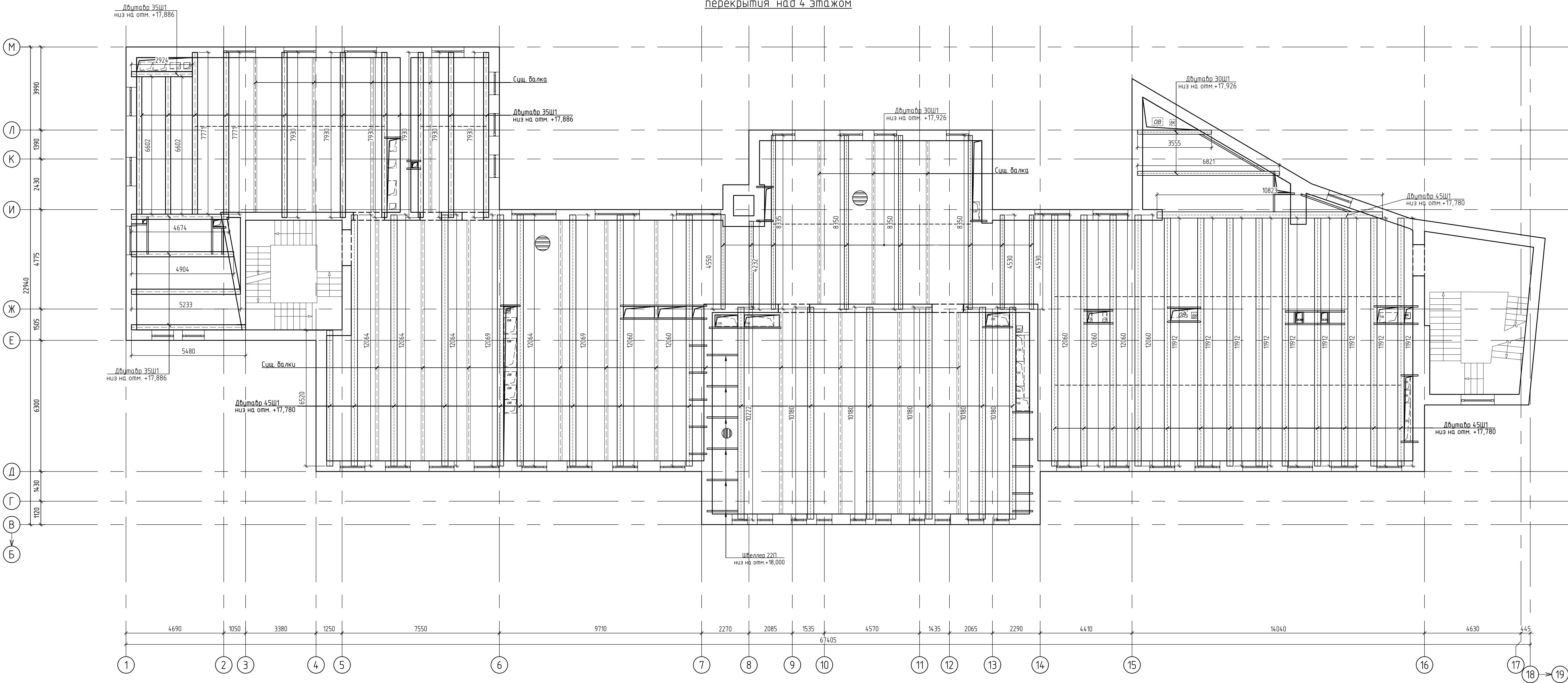
Схема расположения металлических балок перекрытия над 4 этажом
