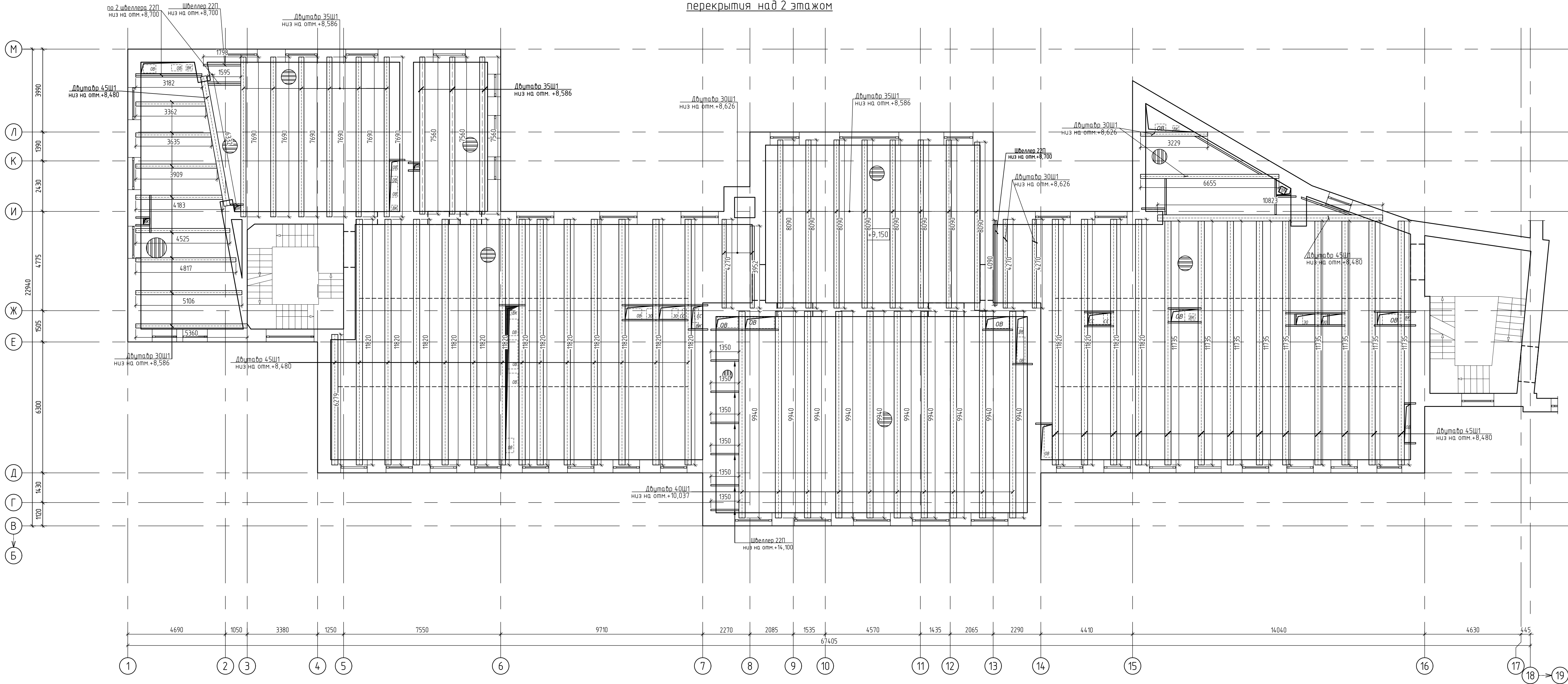
Схема расположения металлических балок перекрытия над 2 этажом
