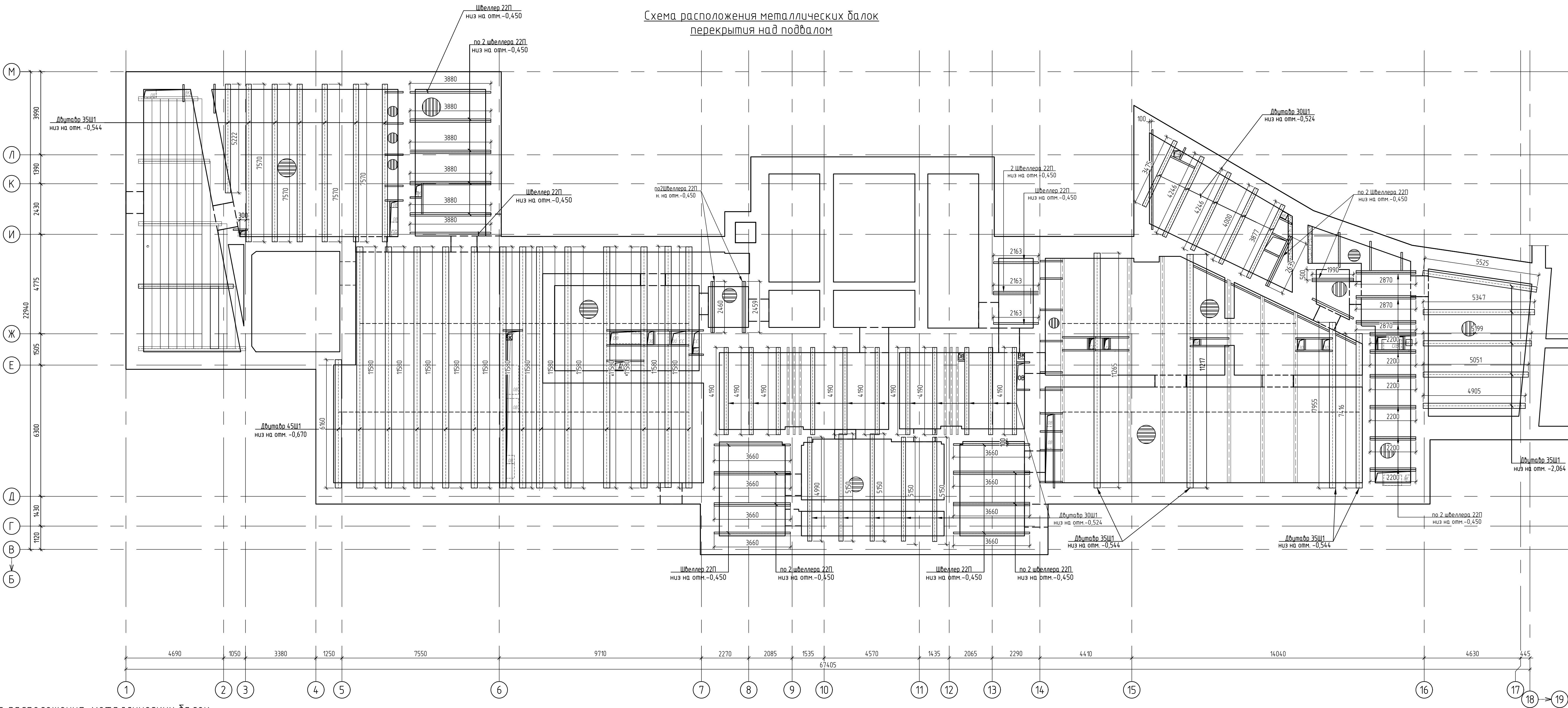
Схема расположения металлических балок перекрытия в осях 9-11 / Ж-Л на отм. -1,050
